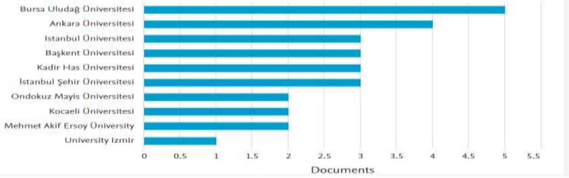
Grafik 4. Kurumlara Göre Akademik Çalışmaların Dağılımı (İlk 10 kurum)
